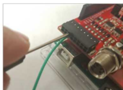
Arduino Shield DI/O アナログ入出力 (4x DI/O +2x アナログ) (DI/O 3-6 番ピン)
